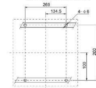
4P: Instalado en rieles delanteros.
