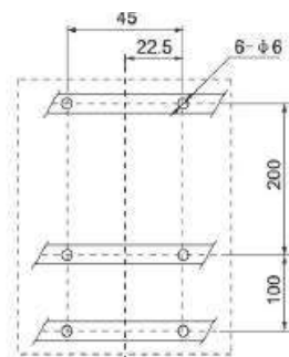
3P: Instalado en rieles delanteros
