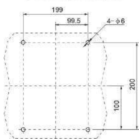
3P: instalado en el panel posterior
