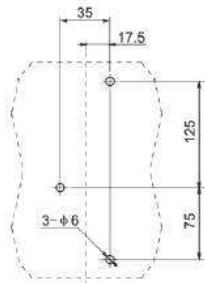
RV20MT-400,630 forma y dimensión
