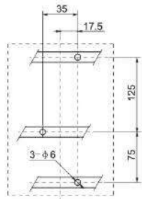
3P: Instalado en rieles delanteros
